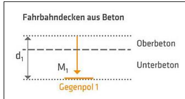
Abb. 12 Dickenbestimmung in Beton
