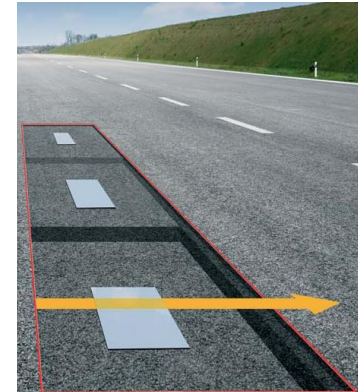
Abb. 12 Messfahrt über einen rechteckigen Reflektor
